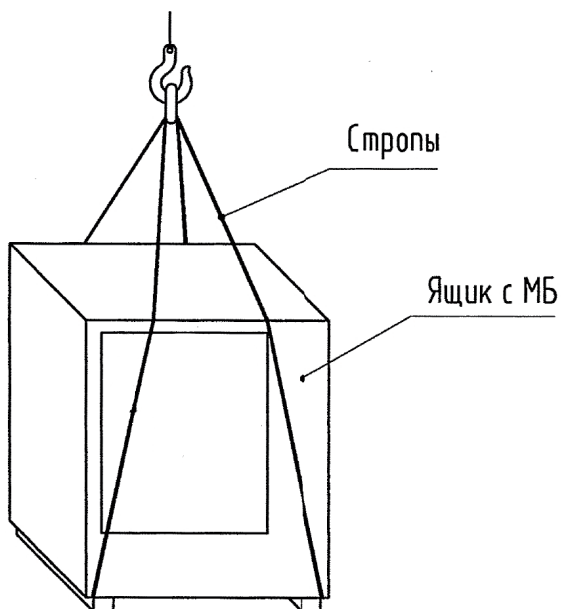
а) Схема подъема мотоблока вручную
