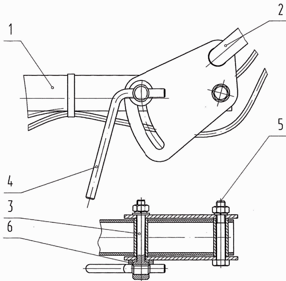
Рис. 9 Регулировка руля.
