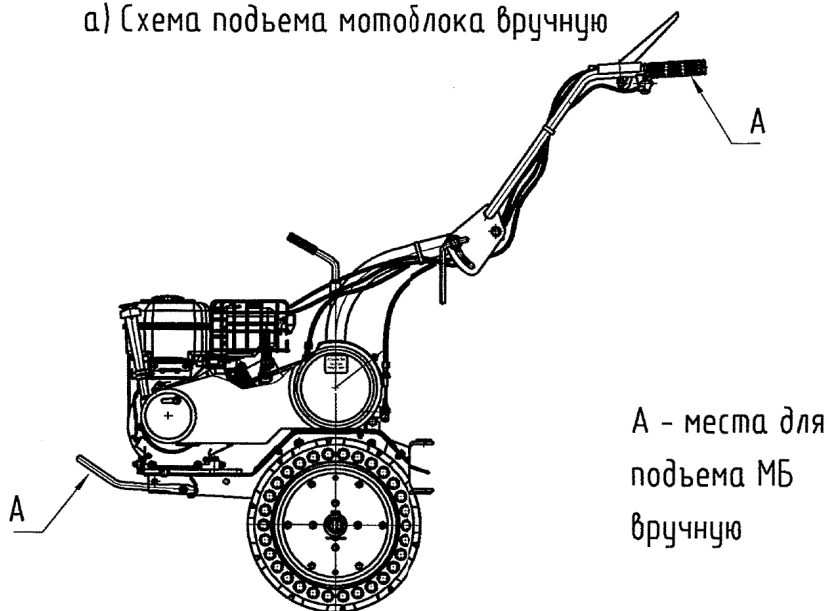
а) Схема подъема мотоблока вручную
